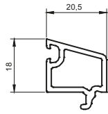
101023 Batiente para vidrio insulado <22mm
