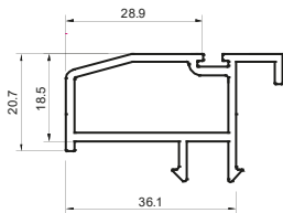
101035 Adaptador de puerta abatible inferior in/out
