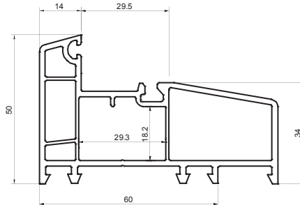
101027 Marco para ventana fija serie 80
