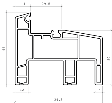
101058 Marco corredizo con fijo integrado
