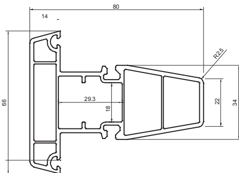
101051 Intermedio para ventana fija serie 80
