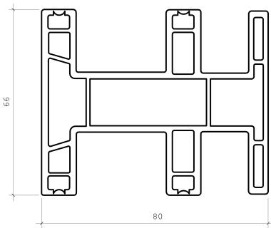
101060 Marco doble corredizo
